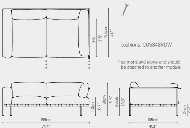
05848RD-x - Right arm corner module 189 cm*
