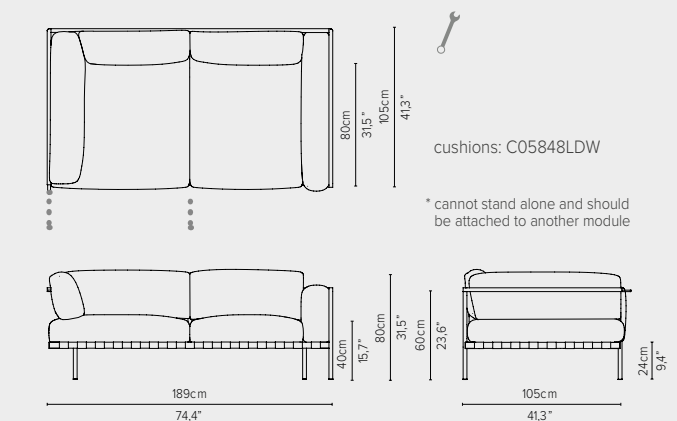
05848LD-x - Left arm corner module 189 cm*
