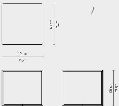
06180 - Coffee table low 40x40cm / 15,75"x15,75"
